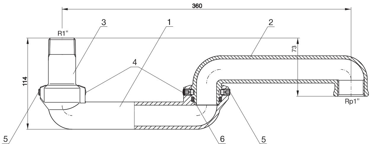
Flexarm® FL 2 (Montage unter dem Rohr) Flexarm® FL 2 (Mounting below the pipe)
